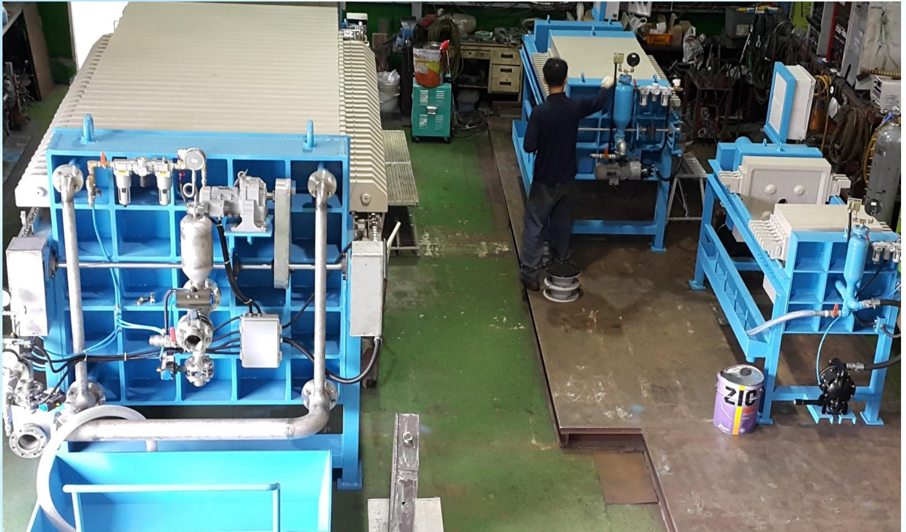
동시 제작중인 폐수처리용 필터프레스 (2000리터, 500리터,1000리터)
